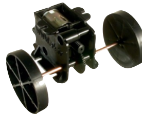
Motor à courant continu Avec réducteur de vitesse par engrenage plastique 4 € l'unité
