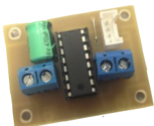
Interface de puissance Pour 2 moteurs à courant continu 5 € l'unité
