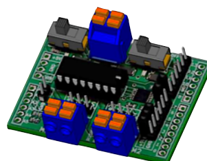
Shield Moteur / Servomoteur Pour 2 moteurs à courant continu ou 2 servomoteurs 10 € l'unité
